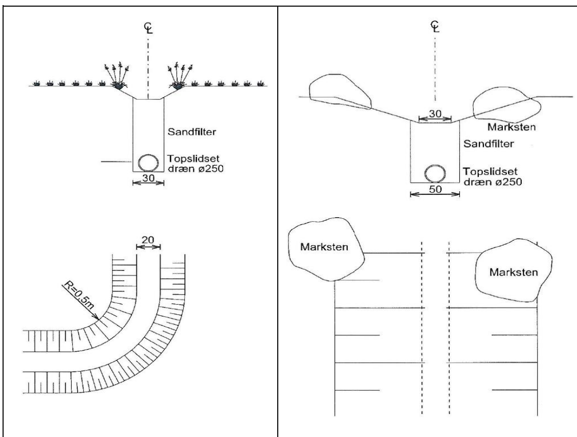
Figur 3.2 Gravede render med sand og grus og opsamlingsrør.
