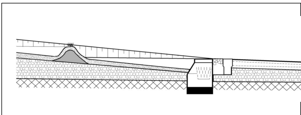
Figur 3.6 Grøft med dæmninger og brønd til neddrosling af udløbet, så der støver vand op i grøften.
