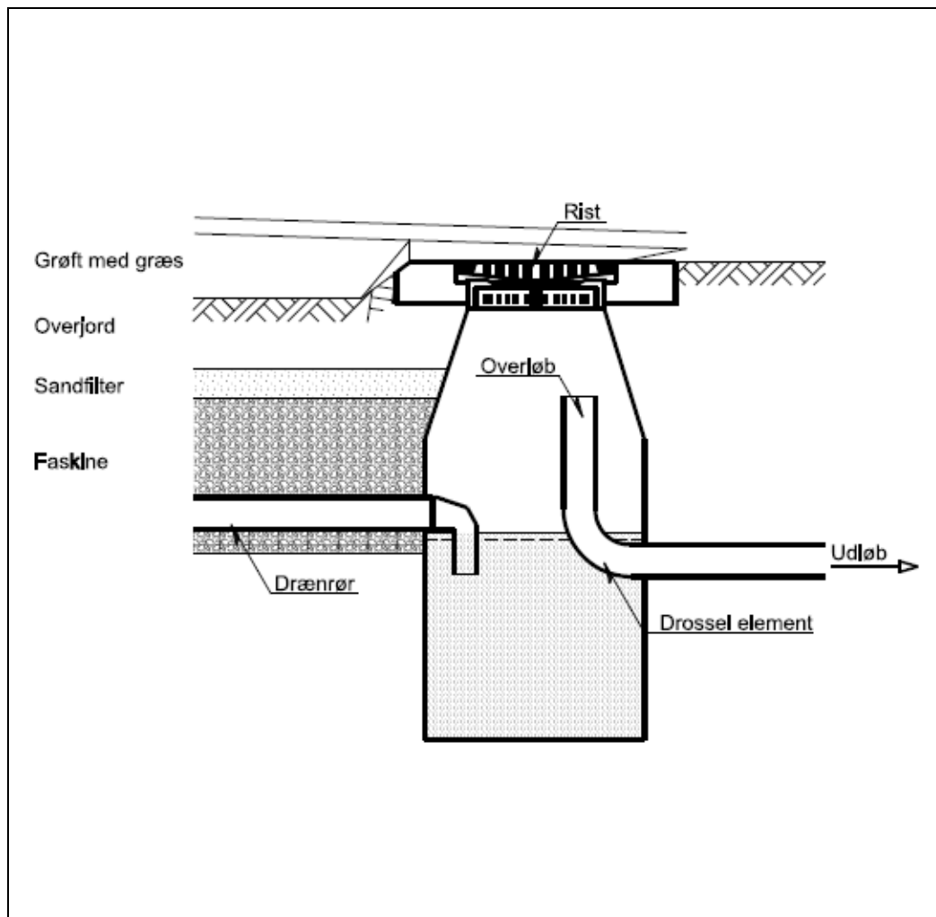
Figur 3.7 Eksempel på neddroslingsbrønd for opstuvning og øget nedsivning af vandet.
