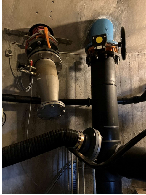
Bundtømmerør
